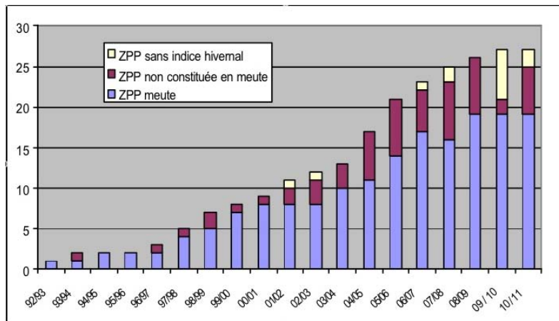
Fig. 7. Evolution du nombre de ZPP de 1992 à 2011. Source: ONCFS (15).
